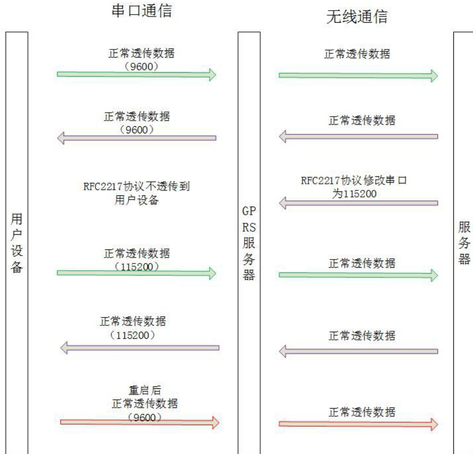
图 10 类 RFC2217 示意图
